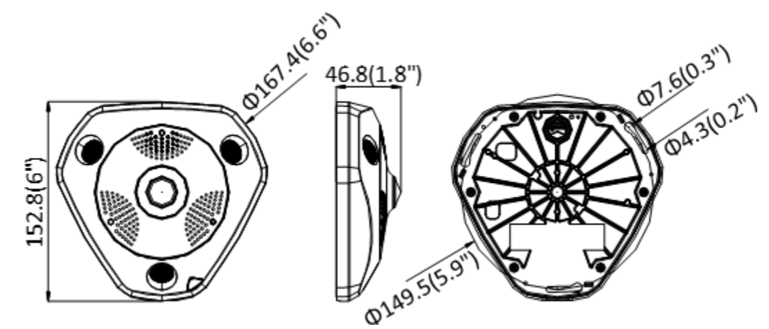
DS-2CD63C5G0E-IS
