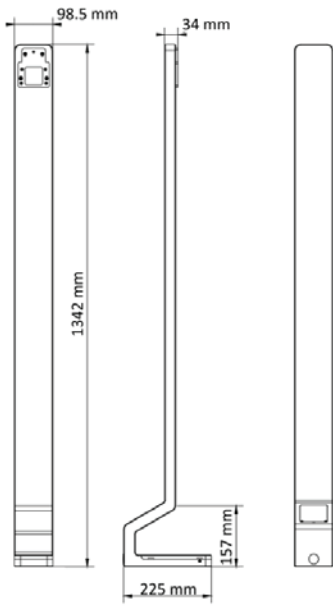
DS-KAB671-B (Optional)
