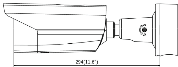
Thermal Bullet
