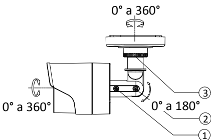
Figura 2. 3 Ajuste de 3 eixos
