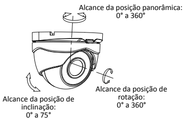
Figura 2. 8 Ajuste de 3 eixos
