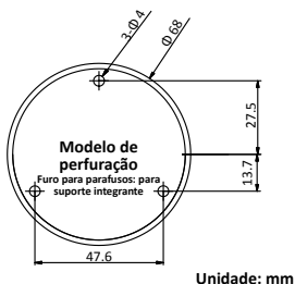
Figura 2. 1 Modelo de perfuração
