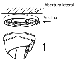
Figura 2. 7 Fixe a câmera na base do suporte de montagem
