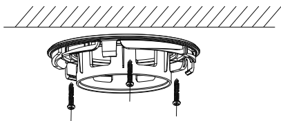
Figura 2. 10 Fixe a base do suporte de montagem no teto
