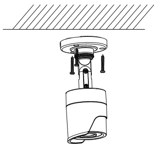
Figura 2. 2 Prenda a câmera ao teto.
