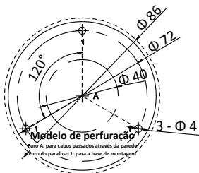
Figura 2. 9 Modelo de perfuração
