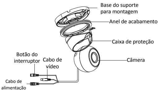
Figura 1. 2 Visão geral da câmera tipo II
