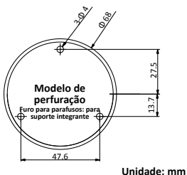
Figura 2. 5 Modelo de perfuração
