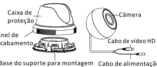
Figura 1-3 Visão geral da câmera tipo III
