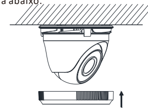
Figura 2-10 Fixação do anel de recorte na câmera
