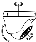
Figura 2-5 Ajuste de 3 eixos
