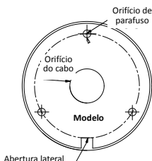
Figura 2-11 Modelo de perfuração
