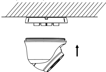
Figura 2-9 Fixe a câmera com o suporte de montagem
