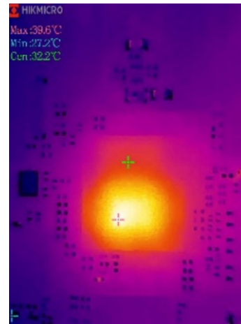
Detecção de placa PCB
