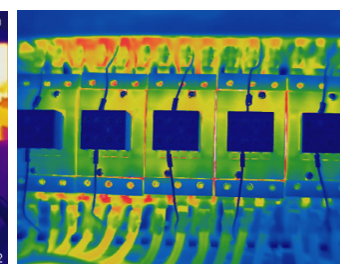
Inspeção de gabinete elétrico
