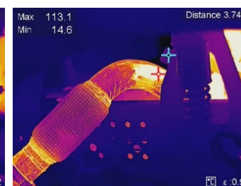
Inspeção de tubulação de óleo
