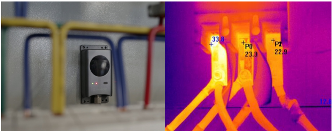
Caixa elétrica
