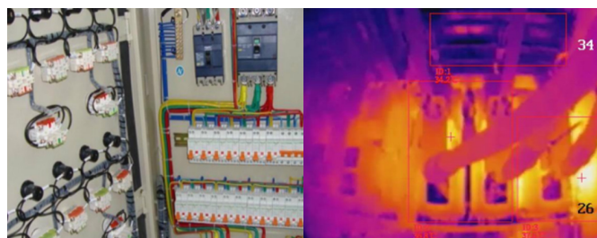
Caixa elétrica
