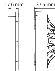
探测器含底座（分解侧视图）
