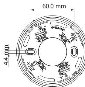
探测器底座（正视图）
