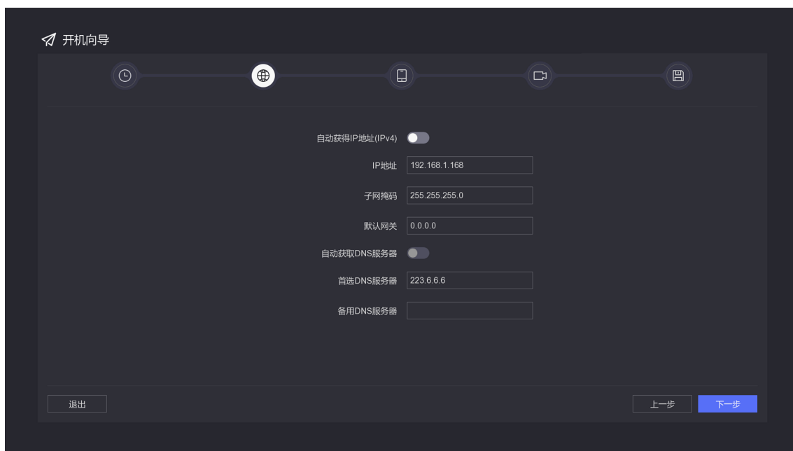
图 2-2 设置网络
