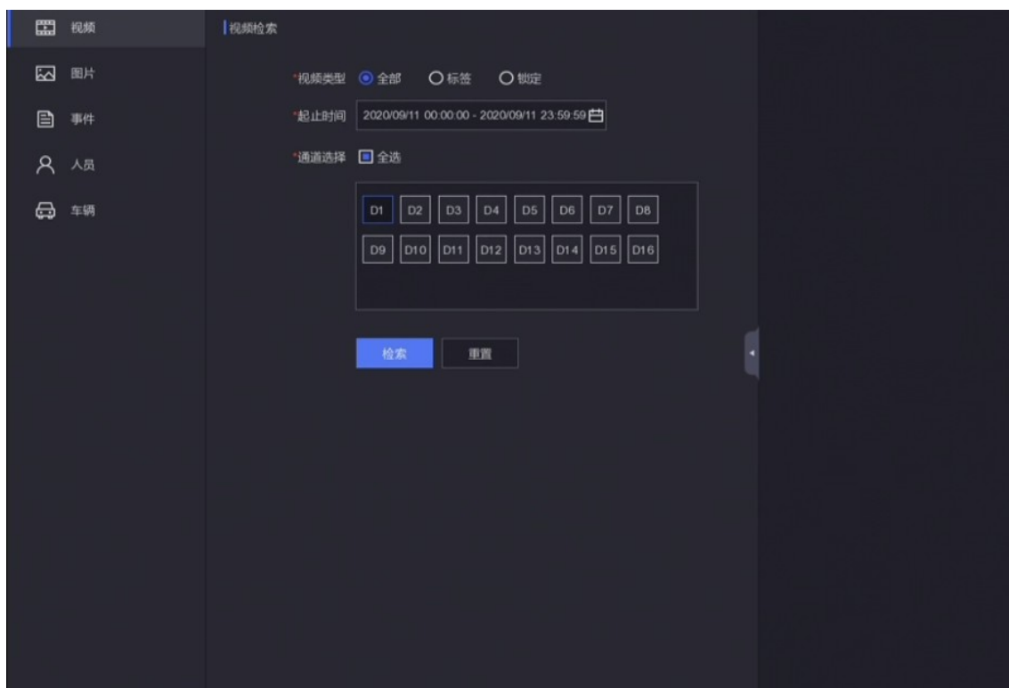
图 7-1 检索界面
