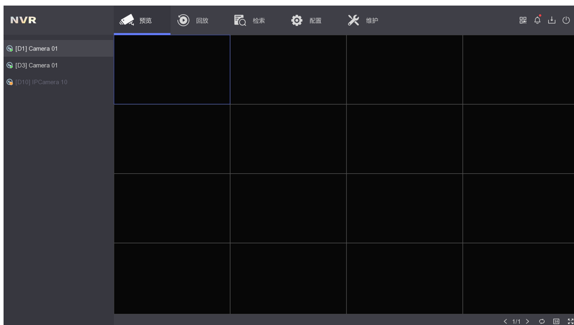
图 5-1 预览主界面
