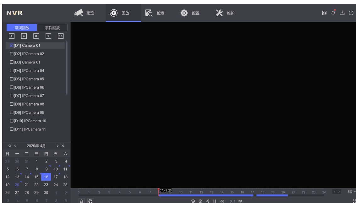
图 6-1 回放主界面
