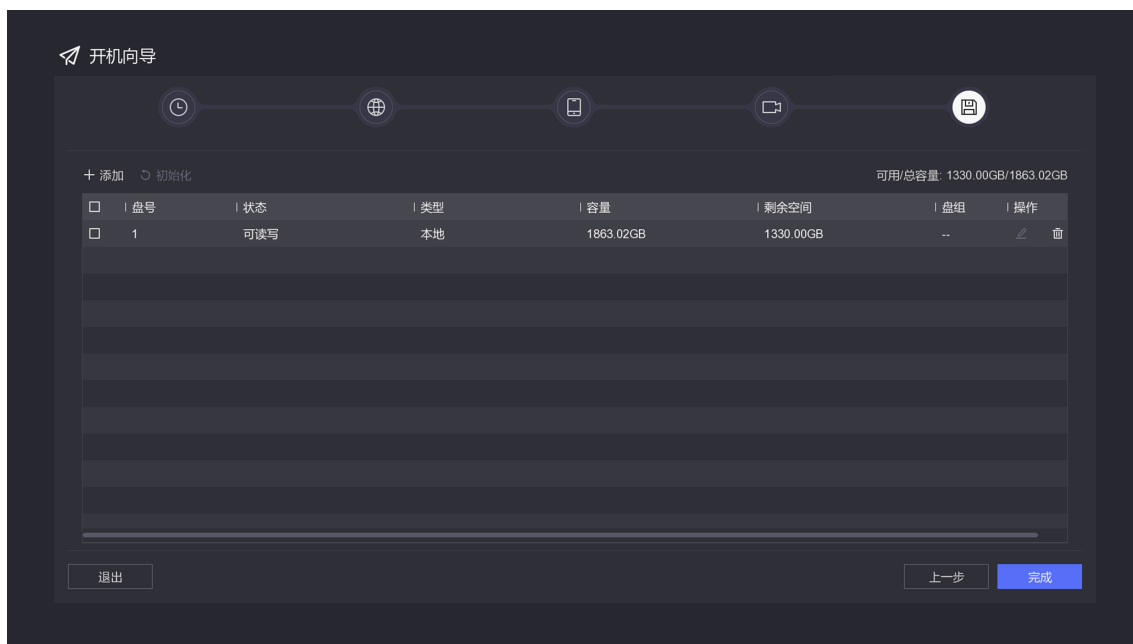
图 2-5 添加硬盘
