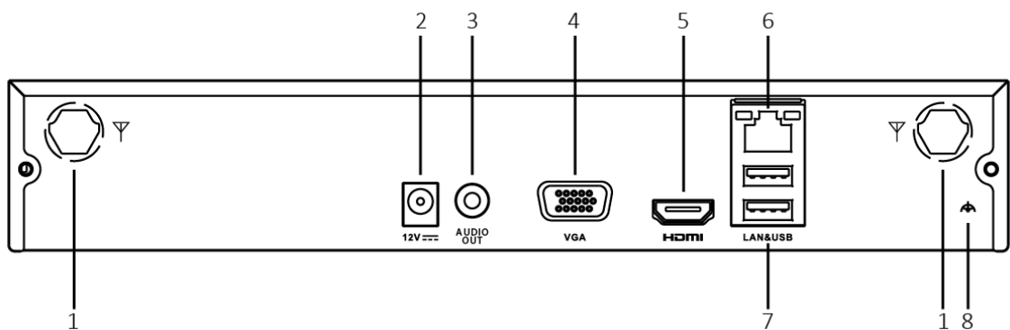
图2-2 后面板示意图
