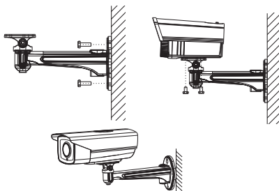
图3-4 筒型摄像机支架安装
