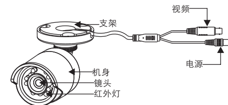
图2-1 I型结构概览
