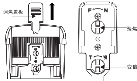
图3-8 调节变倍和聚焦
