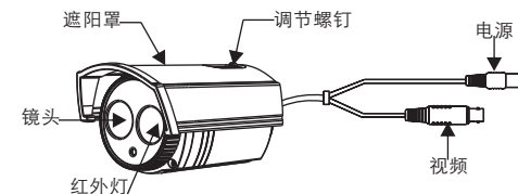
图2-2 II型结构概览
