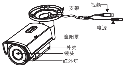
图2-5 V型结构概览
