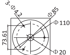
图3-1 安装贴纸
