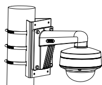
DS-1275ZJ-SUS Montage sur poteau vertical
