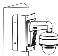
DS-1276ZJ-SUS Montage en angle
