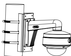
DS-1275ZJ-SUS Montage sur poteau vertical
