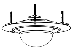
DS-1241ZJ Montage en faux plafond
