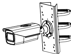
DS-1275ZI-SUS Montage sur poteau vertical
