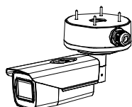
DS-1280ZJ-S Boîtier de jonction
