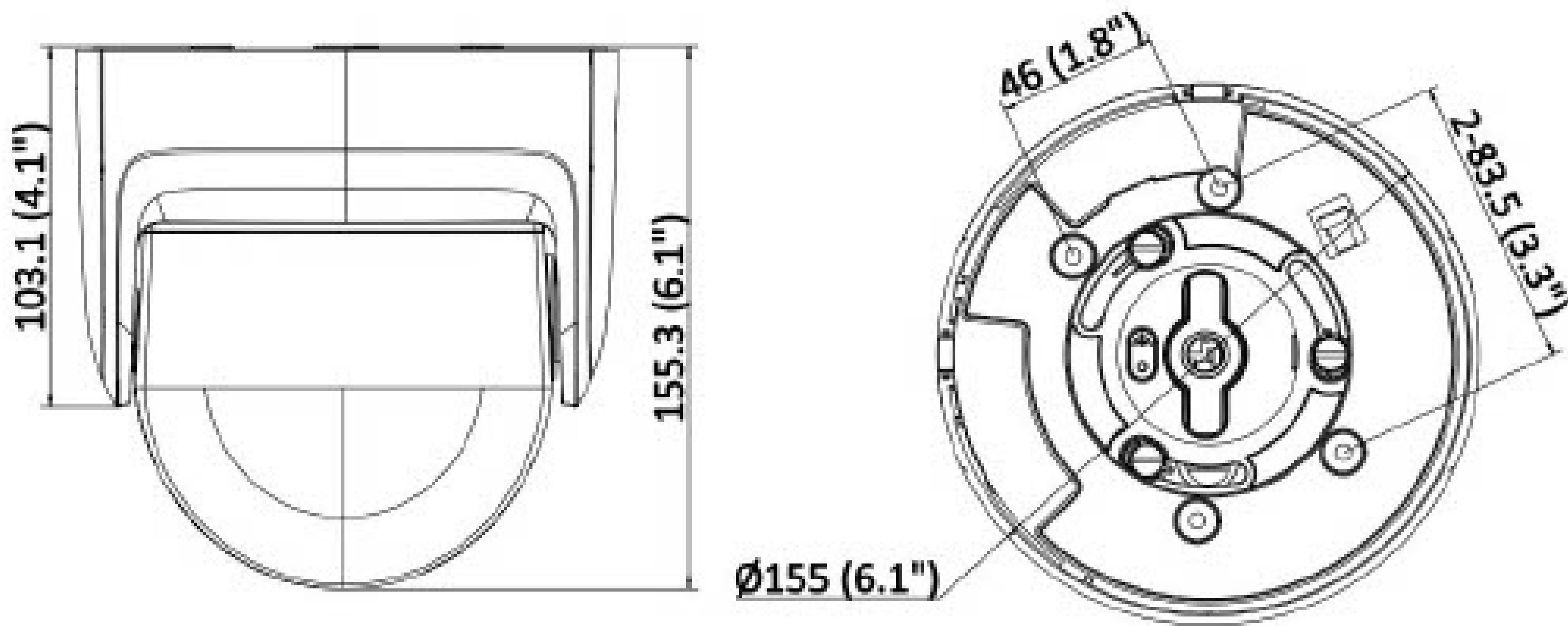
Unit:mm (inch)
